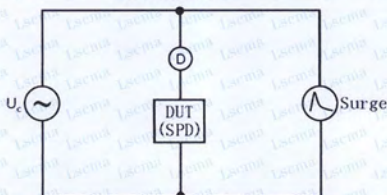
动作负载的测试设置
